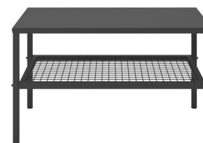
LOV 8 KOD: LOV 0508000005 wys. x szer. x gł. : 502 x 853 x 445 [mm] Stolik z metalowym blatem wykonanym z blachy o grubości 1,5 mm
