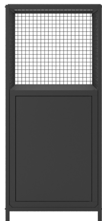
LOV 4A KOD: LOV 0104020202 wys. x szer. x gł. : 1480 x 653 x 445 [mm] Szafka jedno-drzwiowa Sbm 801M Wewnątrz szafki 1 półka
