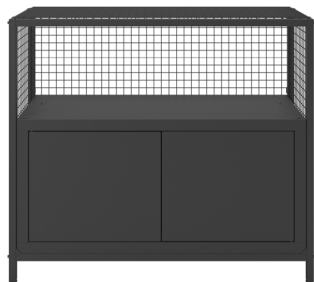
LOV 2C KOD: LOV 0302030202 wys. x szer. x gł. : 910 x 1053 x 44 [mm] Szafka dwu-drzwiowa Sbm 403M Wewnątrz szafki 1 półka
