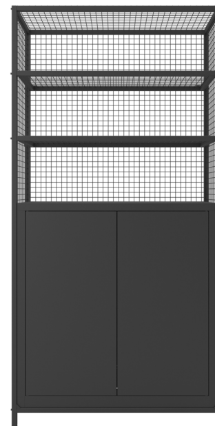
LOV 6C KOD: LOV 0306030304 wys. x szer. x gł. : 2080 x 1053 x 445 [mm] Szafka dwu-drzwiowa Sbm 102M Wewnątrz szafki 2 półki
